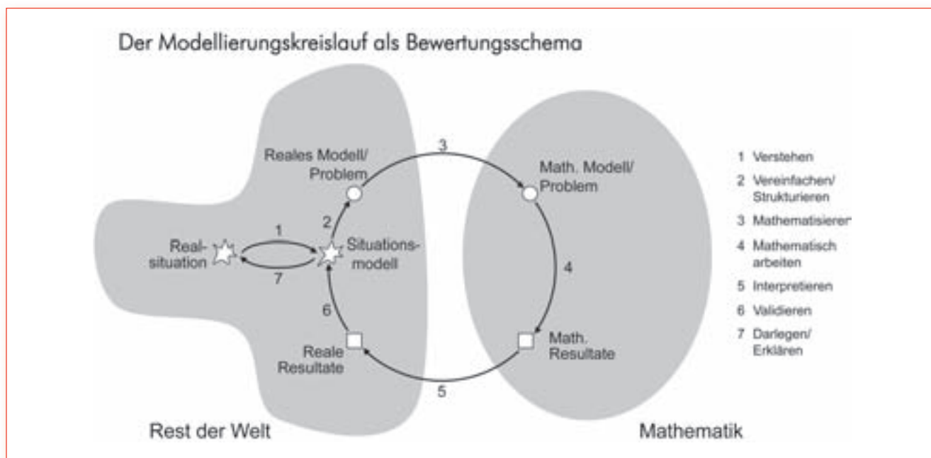
Abb. 1: Modellierungskreislauf (Blum/Leiss, 2005)
