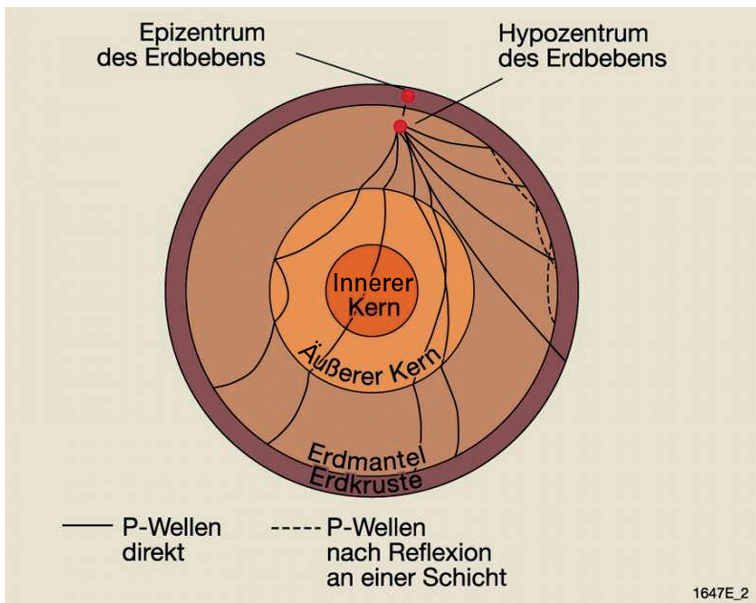
Abb. 3: Verlauf von Erdbebenwellen durch die Erde. Dichteänderungen im Material des Erdkörpers führen zu einer Brechung beziehungsweise Reflexion der Wellen.
